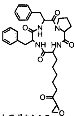
トラボキシシンB
